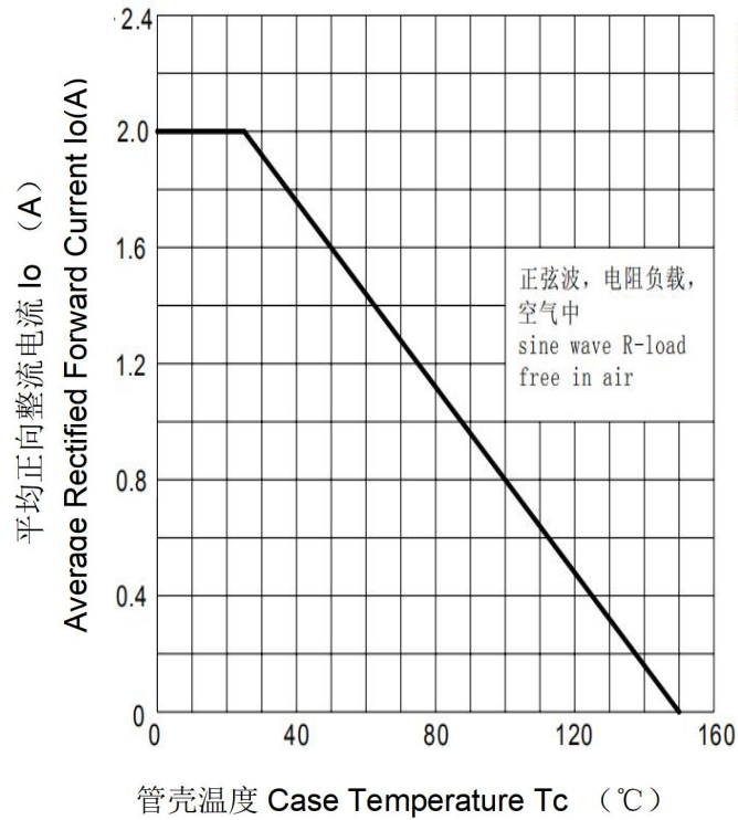
图 1 电流降额曲线 Fig.1: Derating Curve
